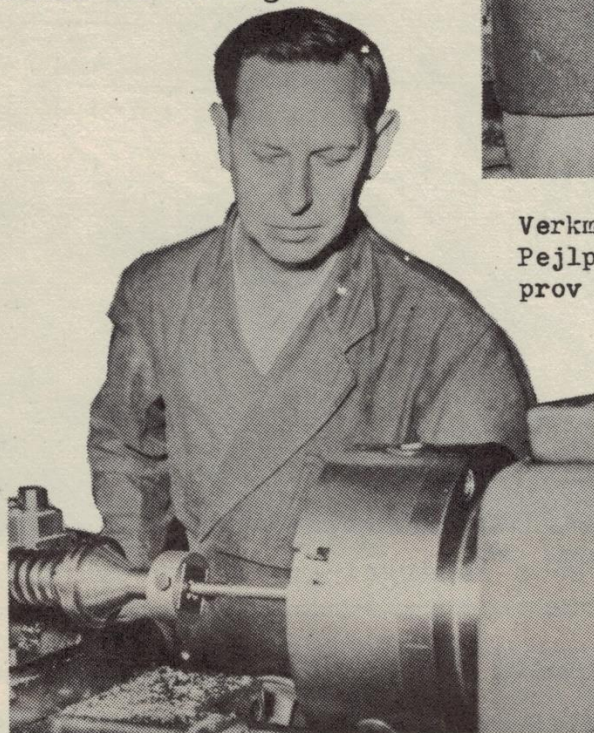
Svarvare Otto Stenmark, Maskinverkstaden: "Anordning så att gängsnitt kan användas i Pearn's gängapparat".
