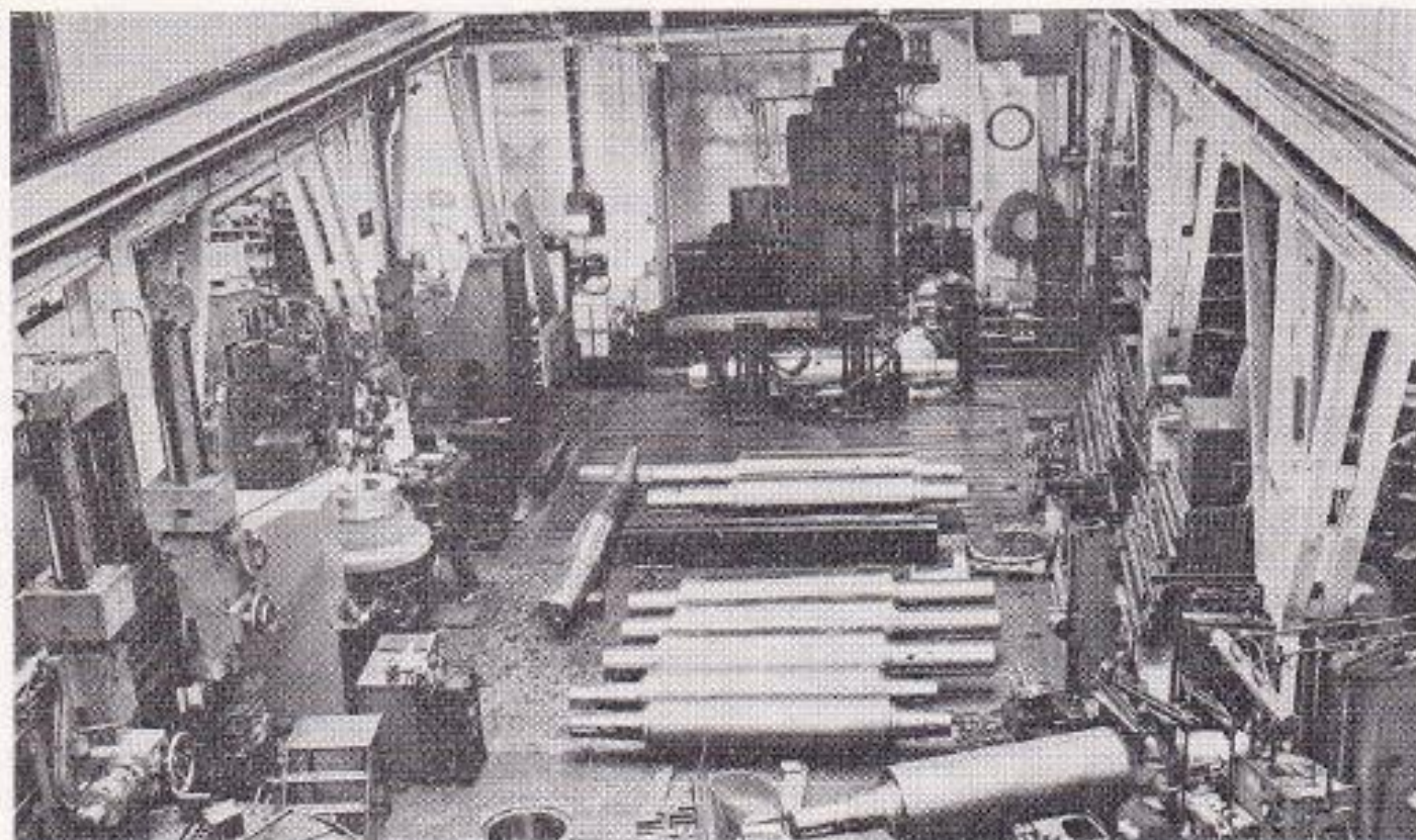
MASKINVERKSTADEN I. De på verkstadsgolvet placerade detaljerna är valsar till drivriktverk.
