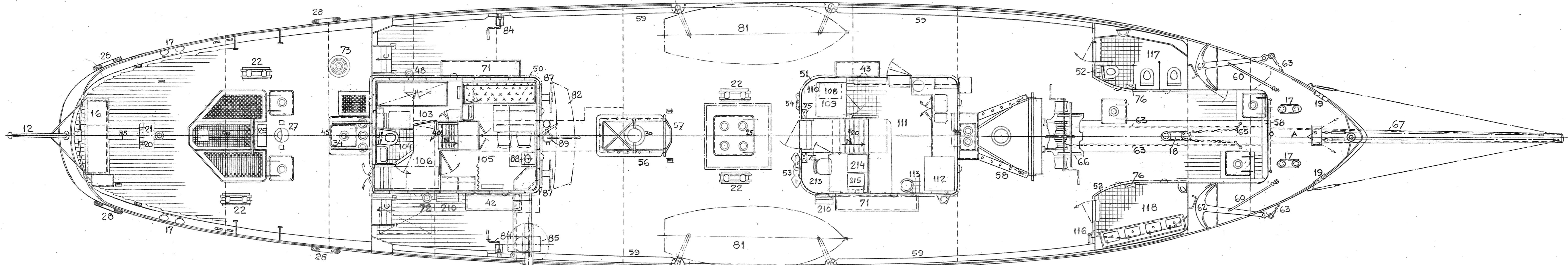
ÖVRE DÄCK.
