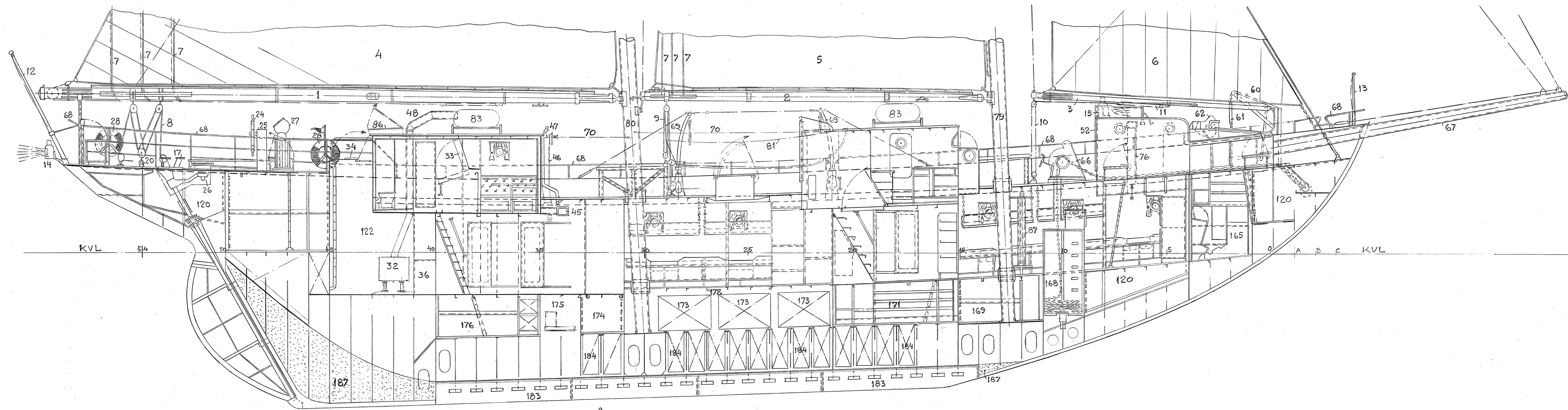
LÅNGSKEPPSSEKTION.
