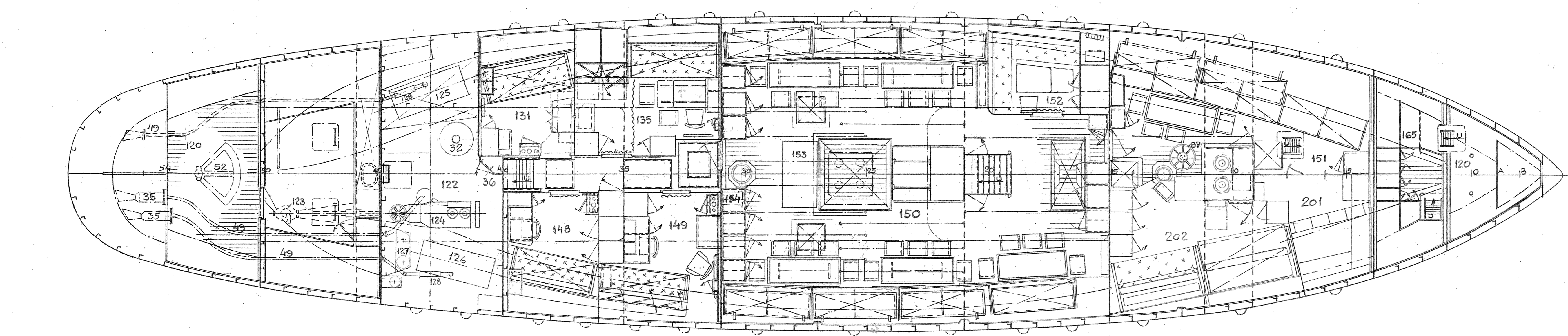
UNDRE DÄCK.
