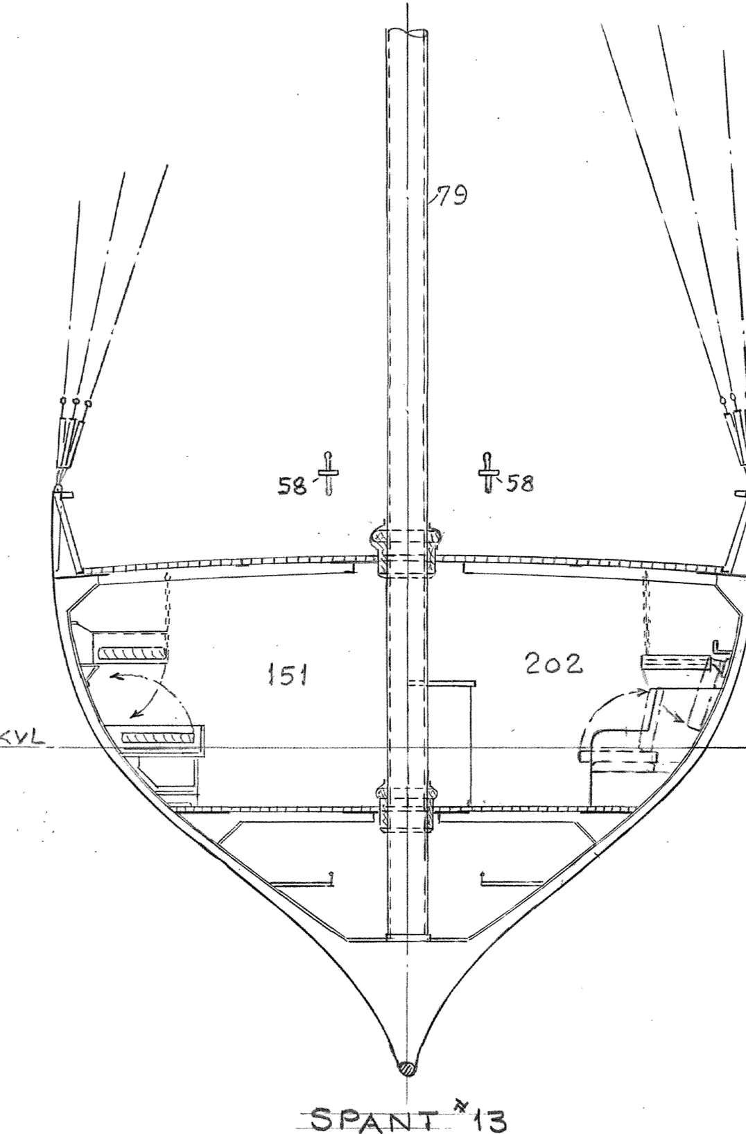
SPANT #13, SETT AKTERIFRÅN.
